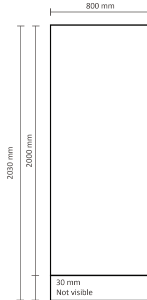
80x200cm (DRUBP1-80)
