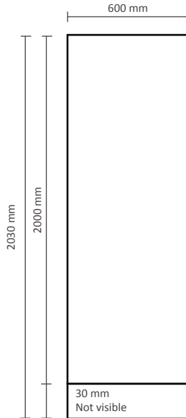
60x200cm (DRUBP1-60)
